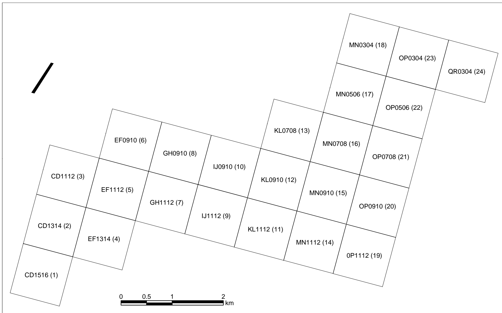
図 4 地図の分割
